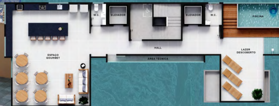
Planta Baixa do Rooftop
